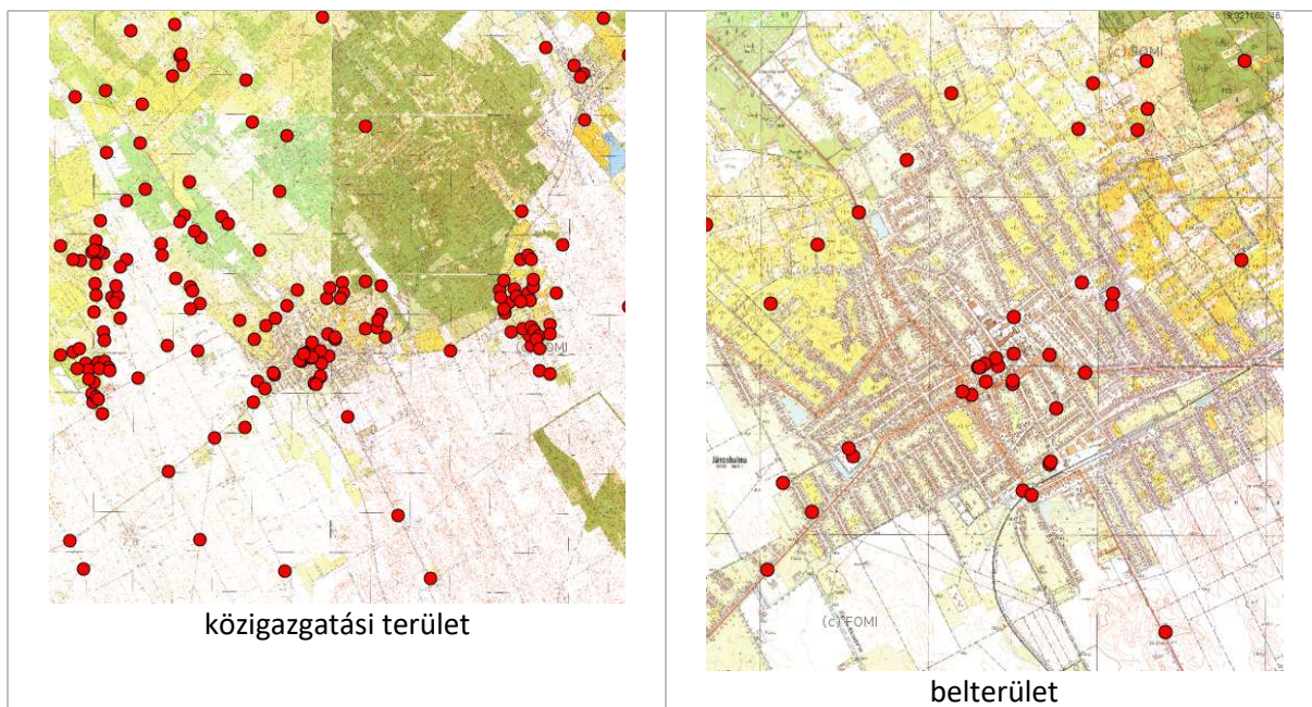
39. ábra: Egyedi tájértékek elhelyezkedése Jánoshalmán
